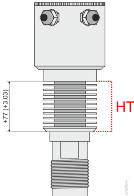
Fig. 3 HT option
